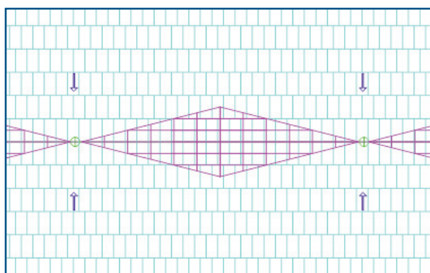
Silka 15: Osnutek postavitve naklona + načrt za montažo
