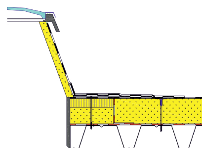
Silka 14: purenit za pritrditev svetlobne kupole
